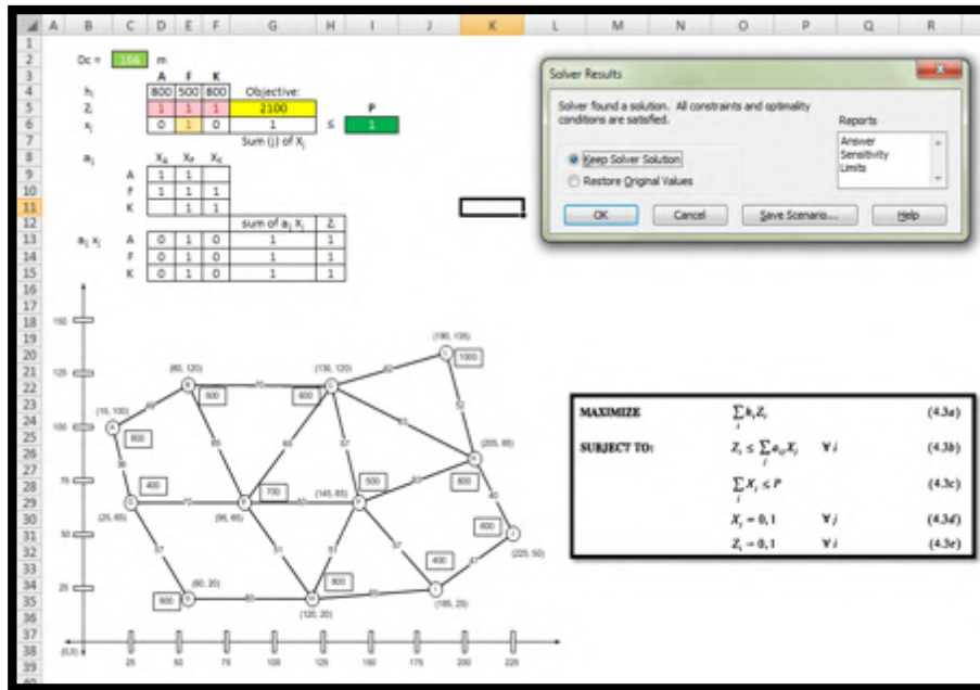
Gambar 10. Screenshot dari Microsoft Solver untuk analisis fasilitas tingkat-2 ( D_c = 166 ).
